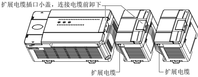
图 5-1 扩展模块级联方法
