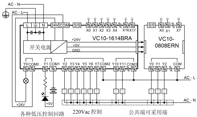
图 4-1 VC10-1614BRA 与 VC10-0808ERN 的电气连接示例
