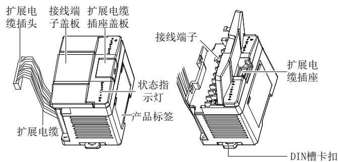
图 1-1 I/O 扩展模块的外形结构与部件
